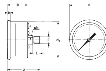
D - POSTERIORE DN50 per montaggio locale.
